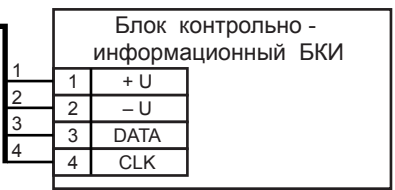
Схема подключения систем громкого оповещения и охраны входов
